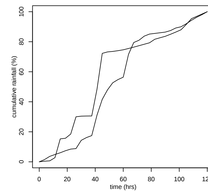
GTSMR swwa_storms 100km 2 120hr
