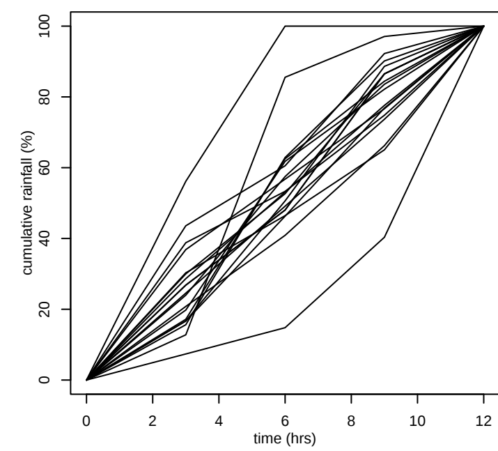
GSAM inland 100km 2 12hr
