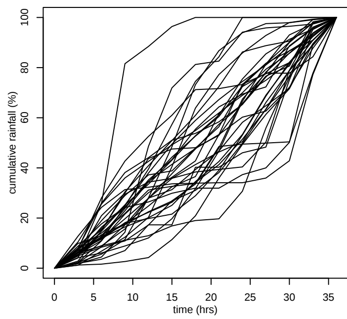
GSAM coastal 500km 2 36hr
