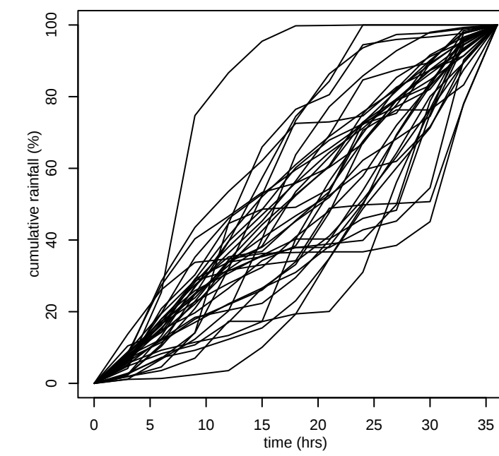
GSAM coastal 1000km 2 36hr
