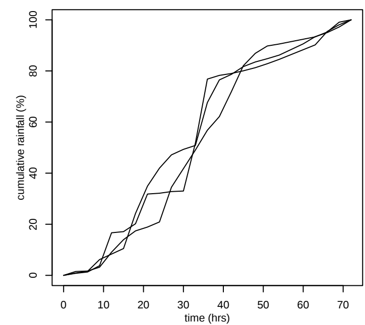
GTSMR swwa_storms 500km 2 72hr
