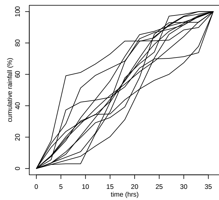
GSAM inland 1000km 2 36hr
