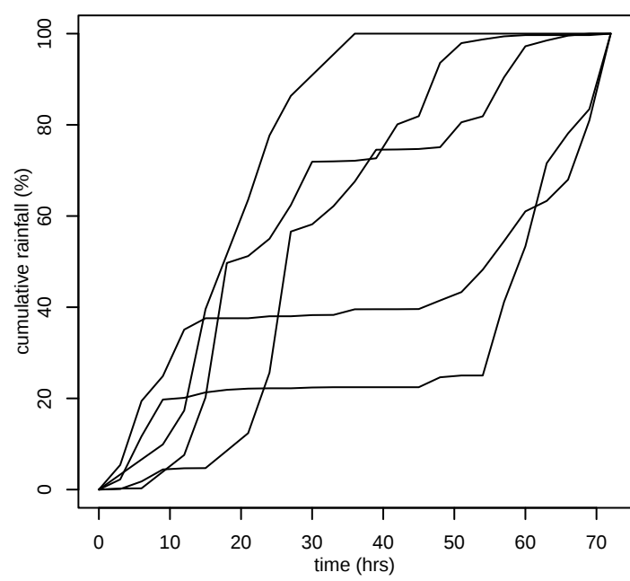
GSAM inland 500km 2 72hr
