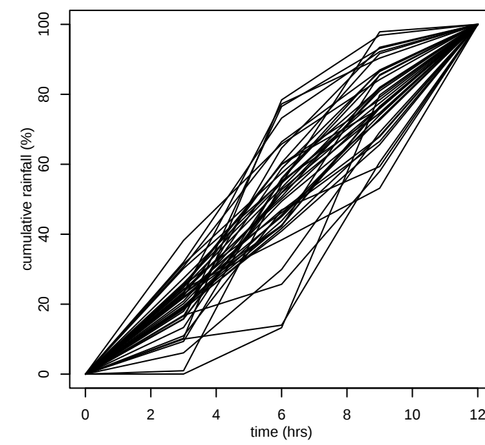
GSAM coastal 1000km 2 12hr
