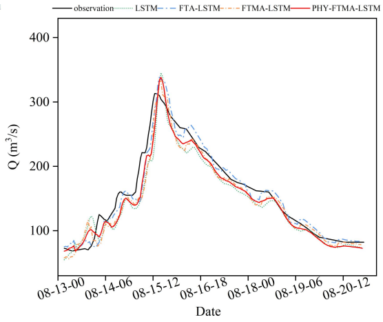
(d) t+4
