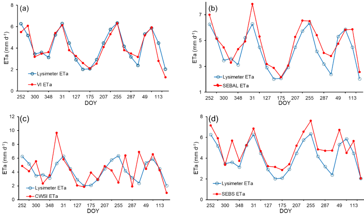
Figure 5. Variability of lysimeter ETa and estimated ETa by VI ETa (a), SEBAL (b), CWSI ETa (c) and SEBS (d) algorithms.
