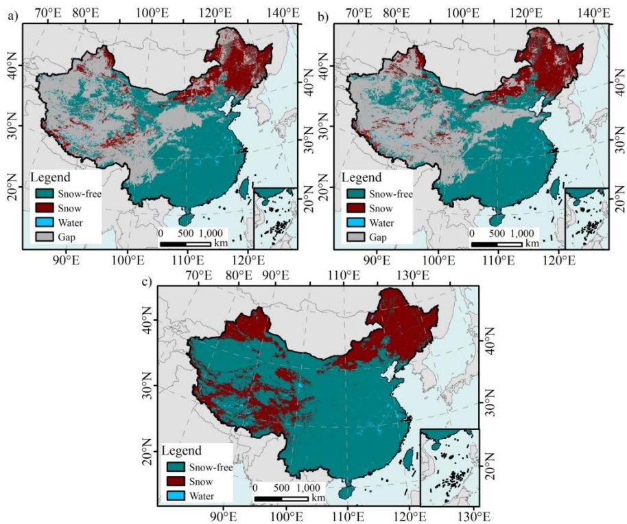
545 Figure 7: NIEER MODIS SCE product on Jan. 4, 2020: a) Terra-MODIS SCE dataset; b) Aqua-MODIS SCE dataset; c) CGF-MODIS SCE dataset
