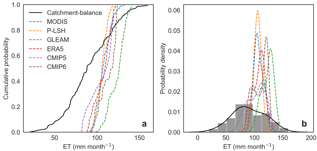
Fig. 1. Kolmogorov-Smirnov analysis
