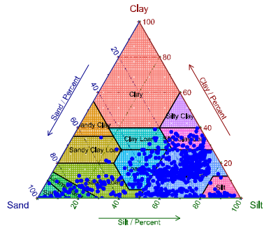
(d) MLP_ILR (63.3%)
