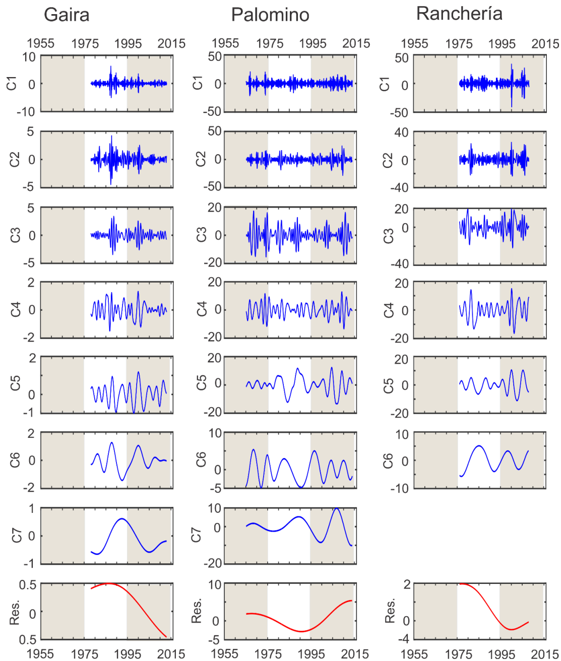
Figure 4. (Cont.) Ensembled Empirical Mode Decomposition (EEMD) for the Fundación, Aracataca, Frío, Gaira, Palomino and Ranchería Rivers.
