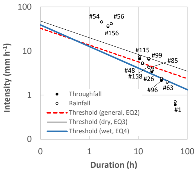
(d) Large events
