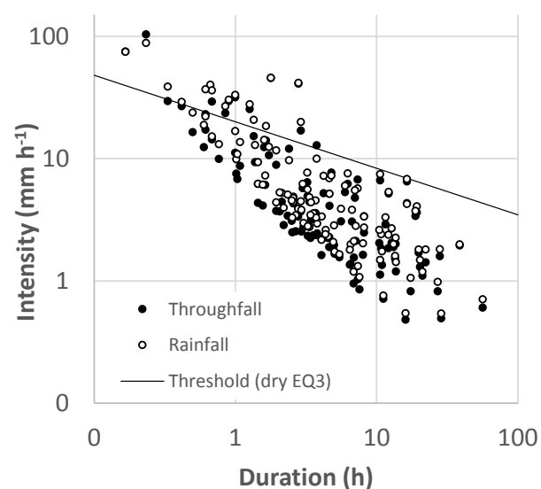
(d) Large events
