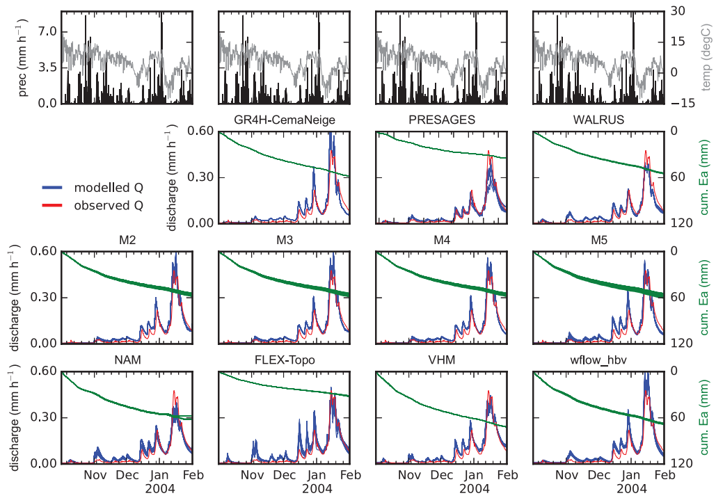
Figure 30: Semois at Membre
