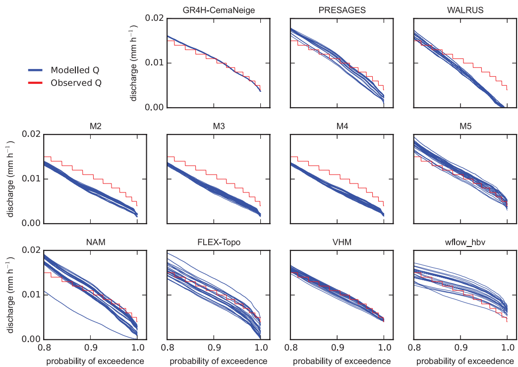
Figure 20: Semois at Membre
