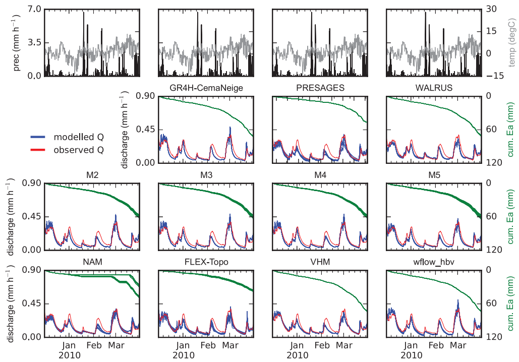
Figure 40: Semois at Membre
