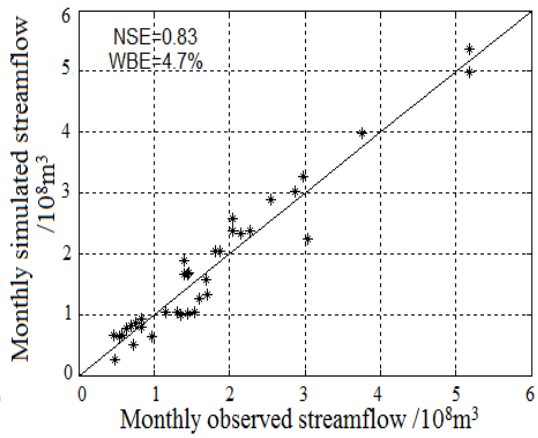
(d) validation streamflow for VIC model
