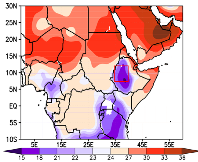
b) RegCM-CRU Temp. at 2m (Celsius)
