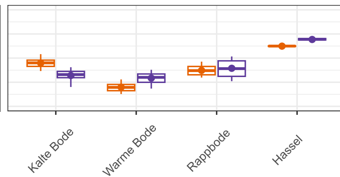
(d) KGE (Landscape-explicit)
