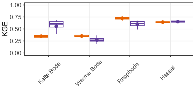
(c) KGE (Lumped)
