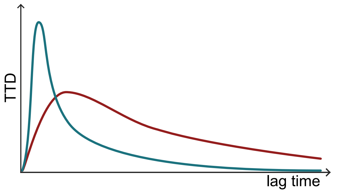
(d) Travel time distributions (TTD)
