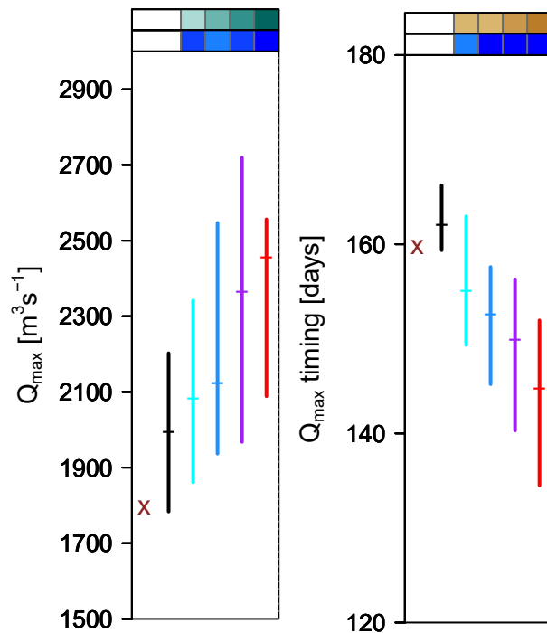
(d) Liard-UC: CWatM
