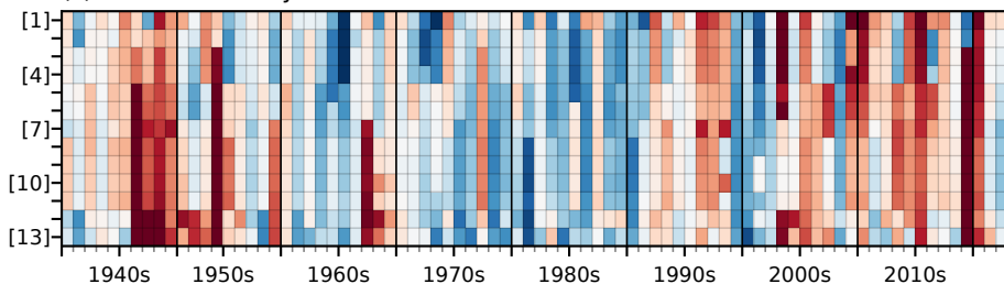
(d) Dam impacts on wet season onset
