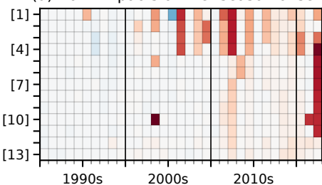
(d) Dam impacts on wet season onset
