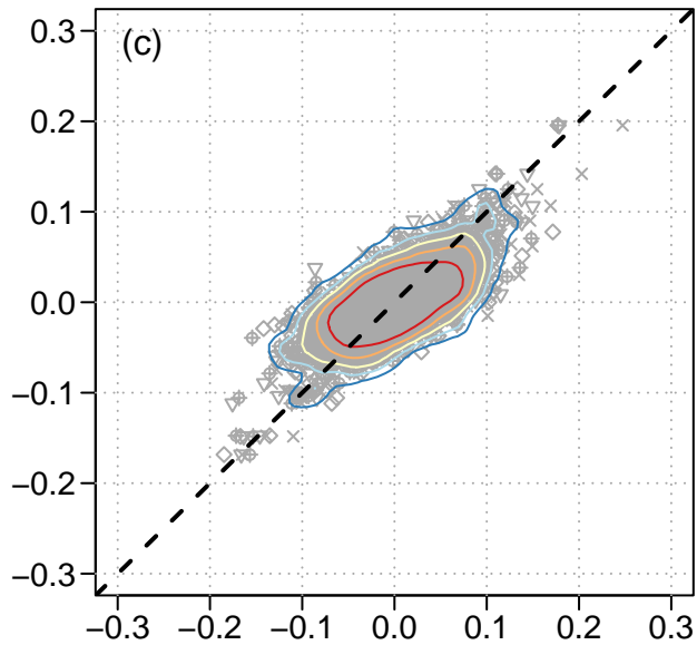
IAAFT
