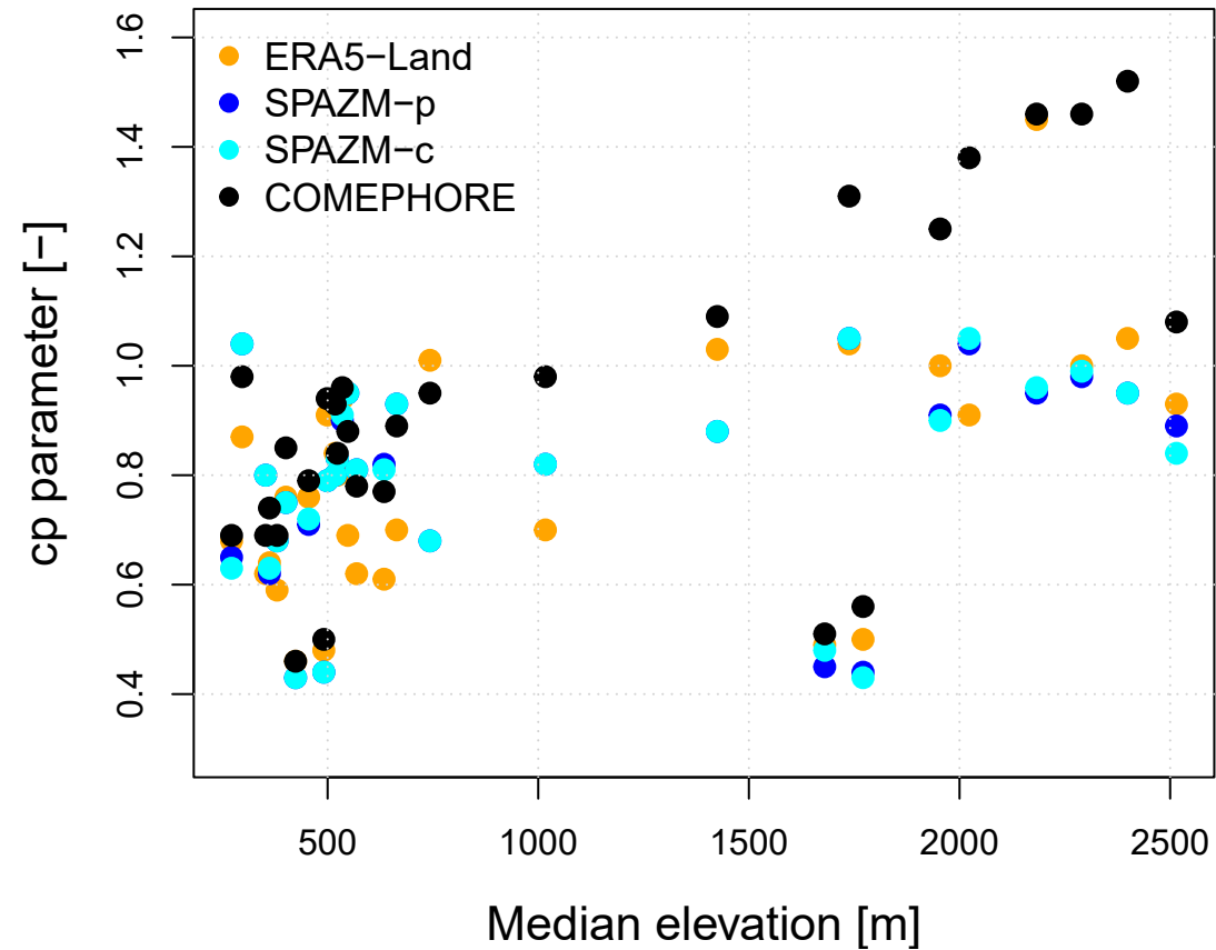
(b) cp parameter versus elevation
