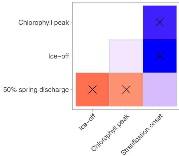
SSP5-8.5
