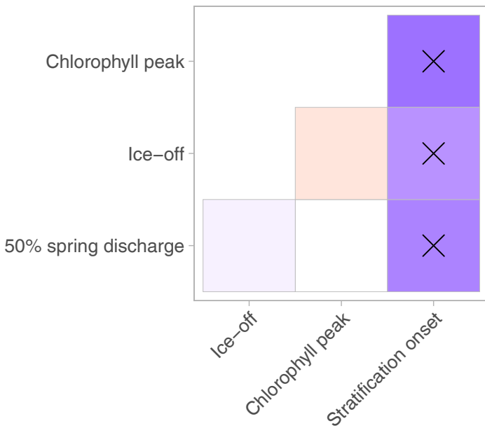
SSP2-4.5
