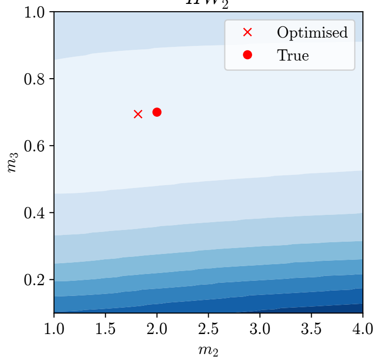
HW_2^2
