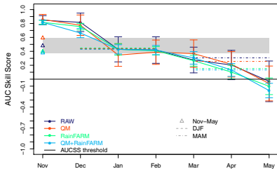
ecmwfS5 AUCSS Lower Tercile
