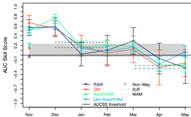
mfs6 AUCSS Lower Tercile
