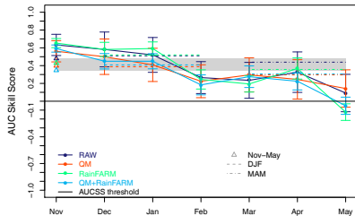
ecmwfS5 AUCSS Upper Tercile
