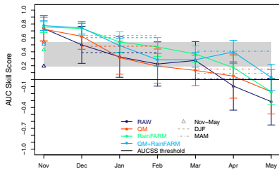
mfs6 AUCSS Upper Tercile
