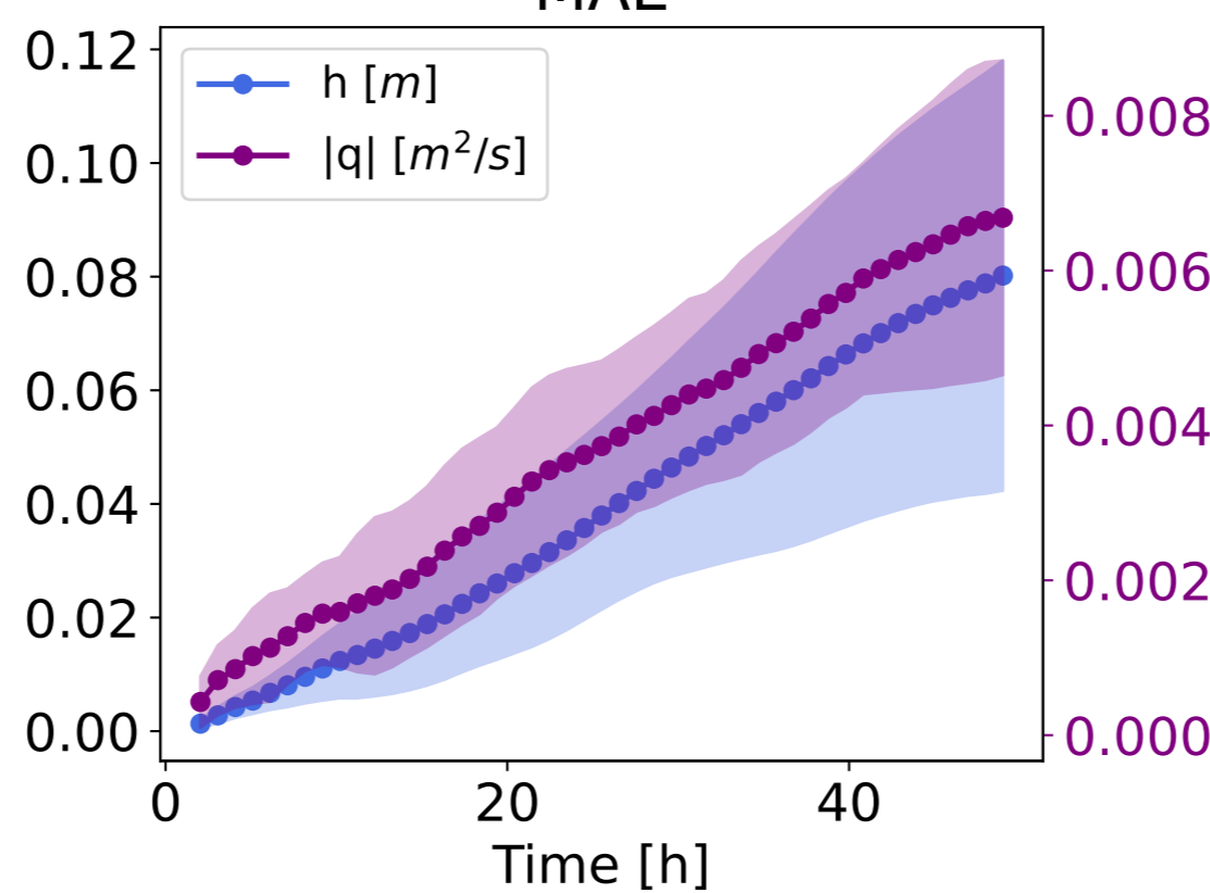
MAE
