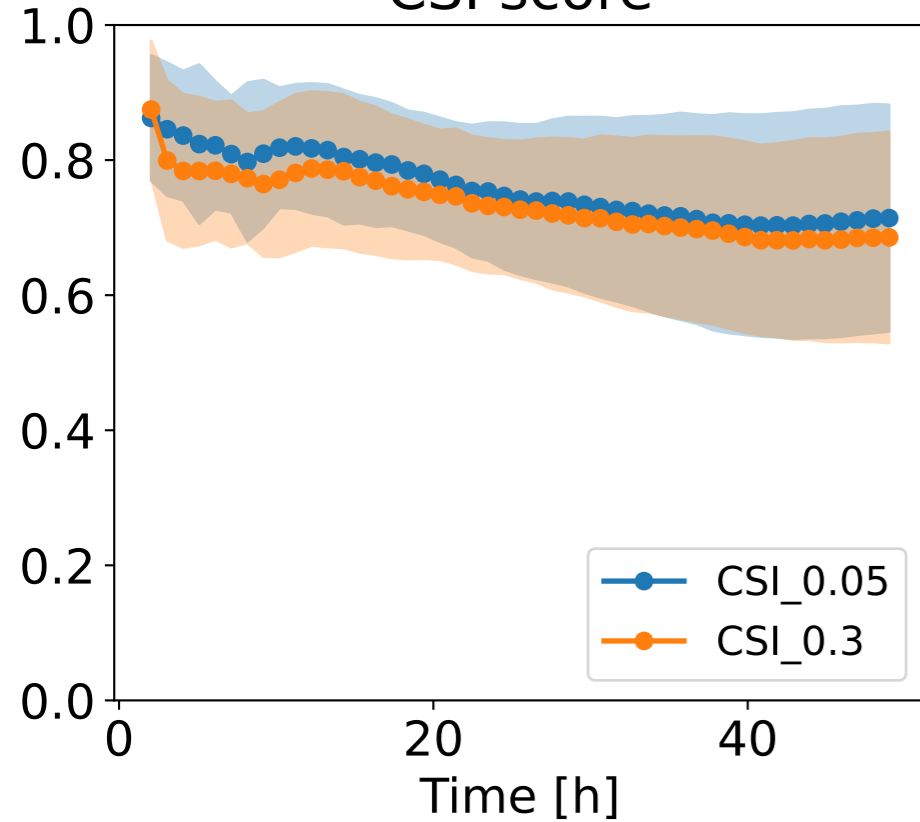
CSI score
