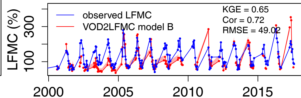
(d) Site with percentile 95% of KGE
