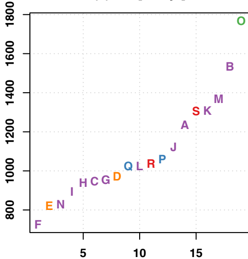
(d) PA [mm/yr]
