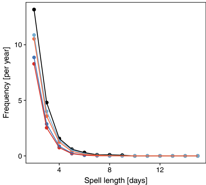
(b) Areal Wet Spells
