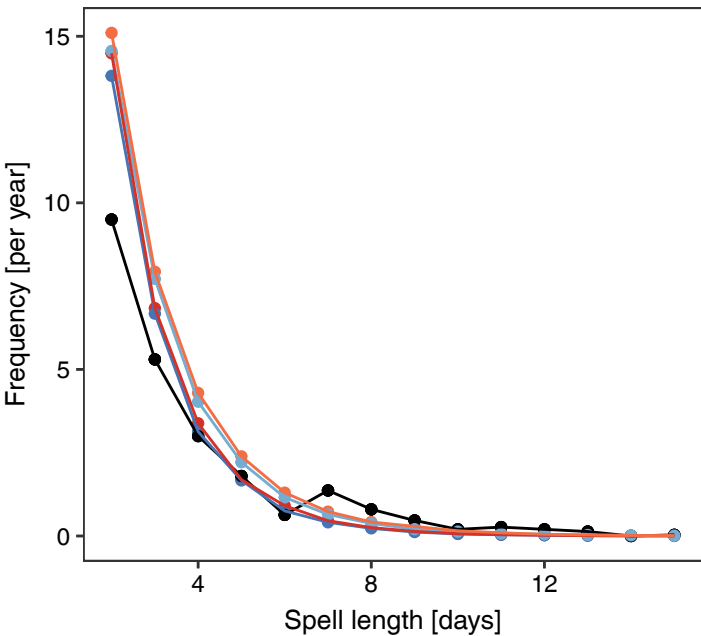
(a) Areal Dry Spells
