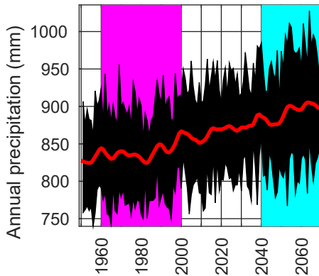
(d) Rainfall
