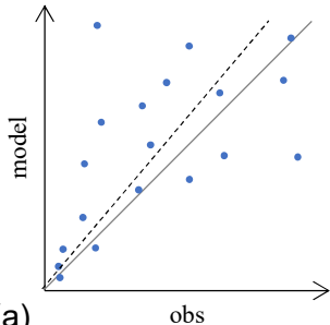
Linear regression
