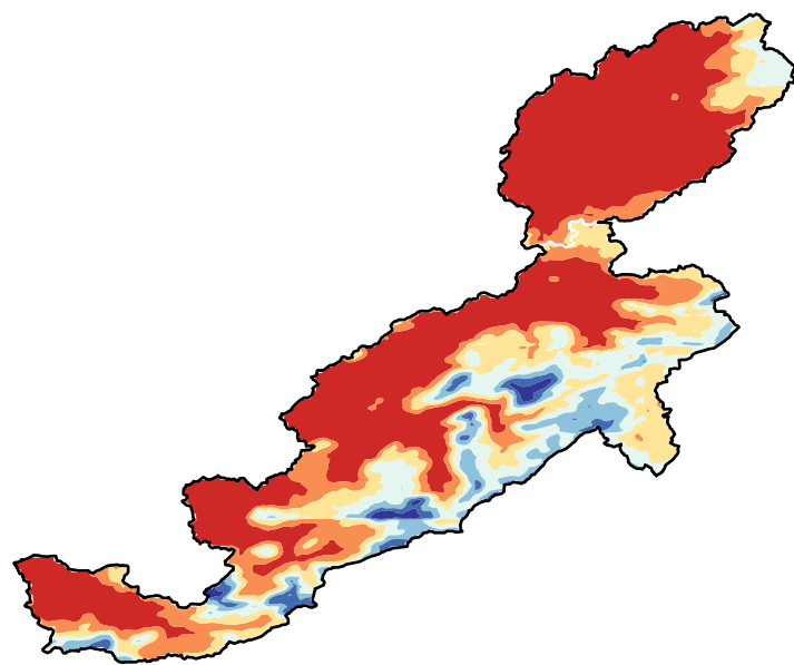
(d) (IPSL-CM5A-LR, 1976-2005)
