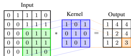
(d) Convolution operation
