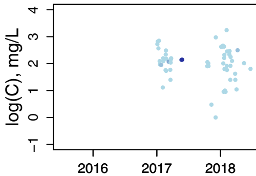
TROPa BFI_m = 0.03 BFI_range = 0.09
