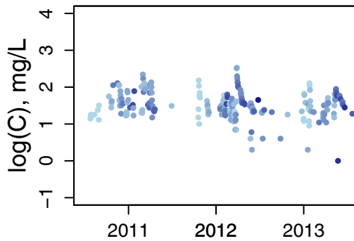
TROPb BFI_m = 0.22 BFI_range = 0.48
