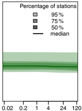
(d) monthly d-GEV
