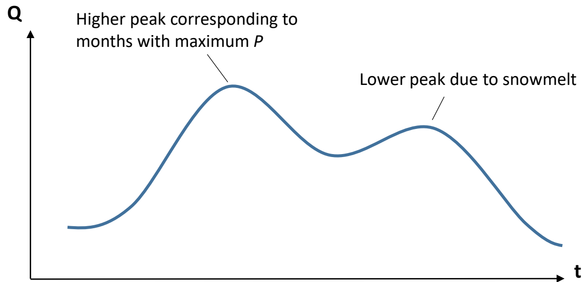
Pluvio-nival
