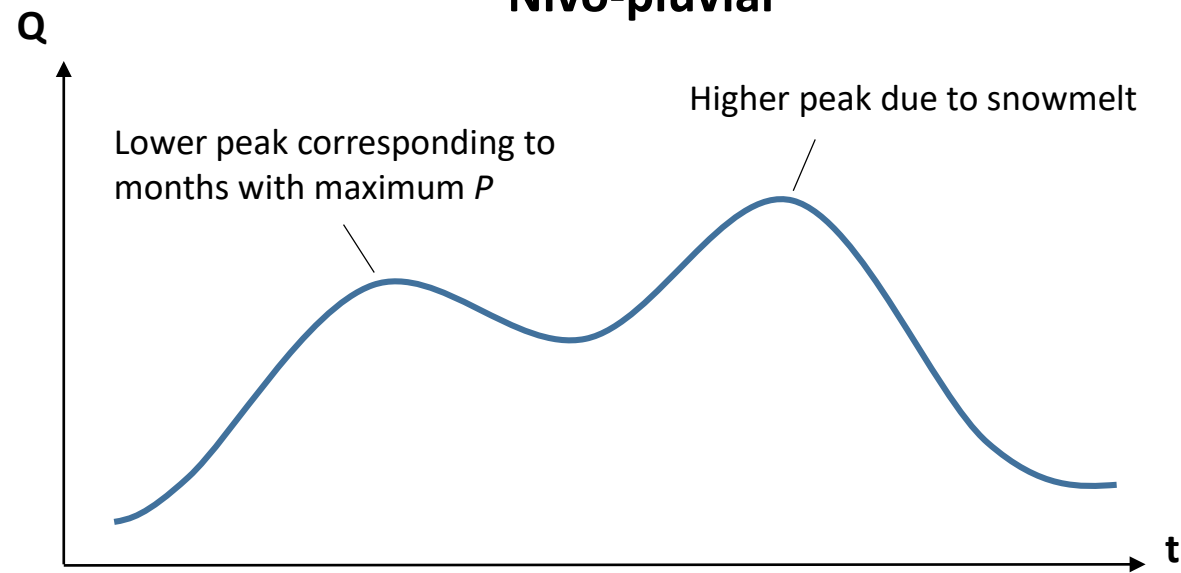
Nivo-pluvial
