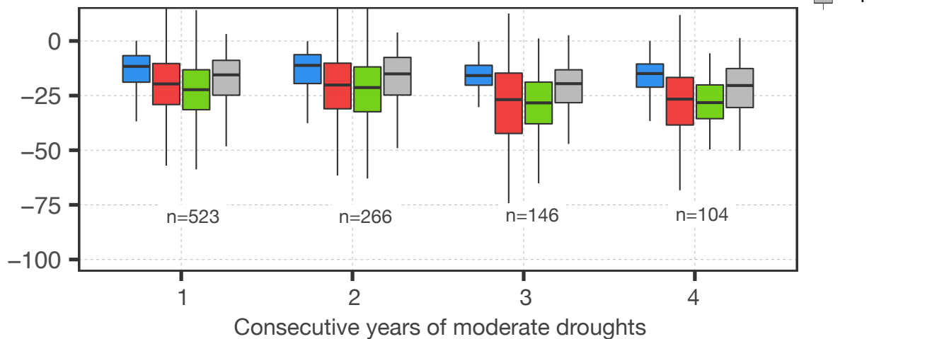
(d) Moderate & mild droughts Pluvial catchments
