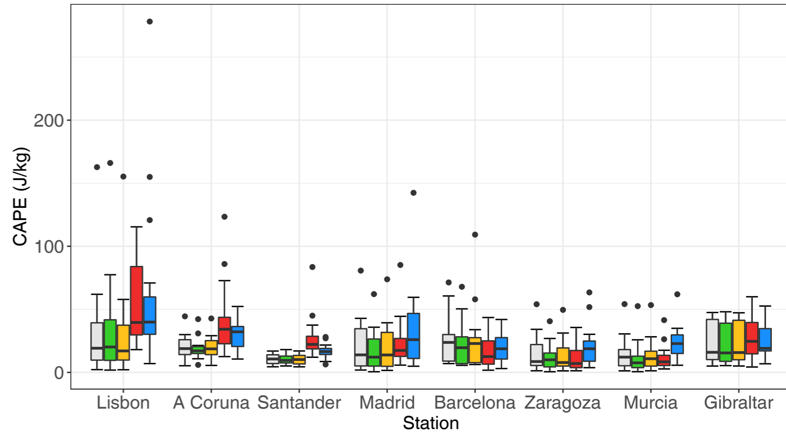
(b) CAPE – Spring MAM (Monthly data)
