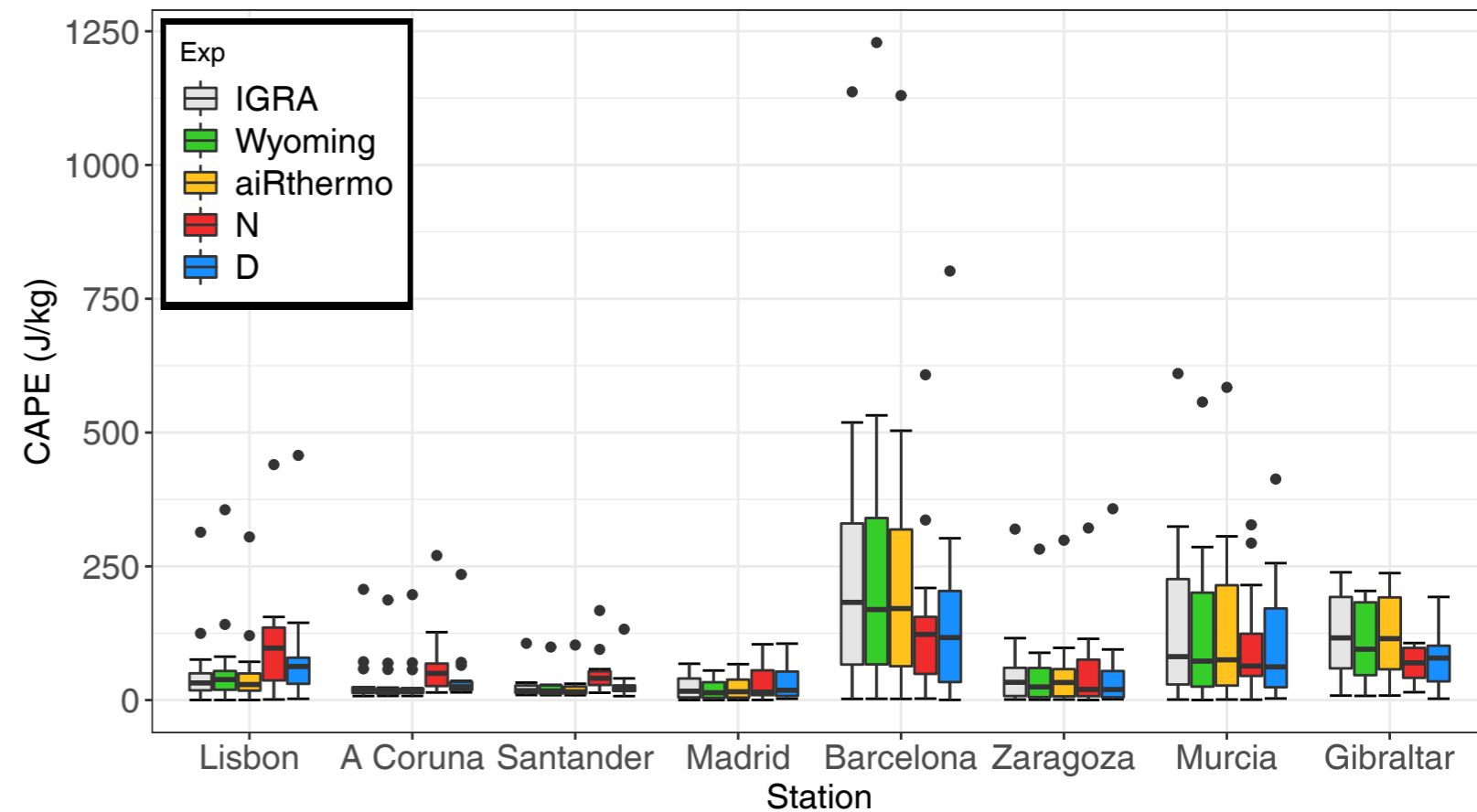
(d) CAPE – Autumn SON (Monthly data)
