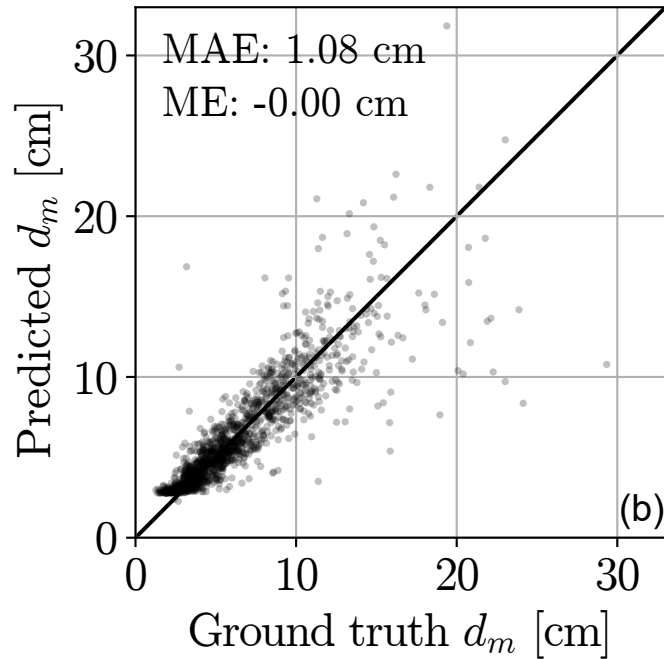
GRAINet volume
