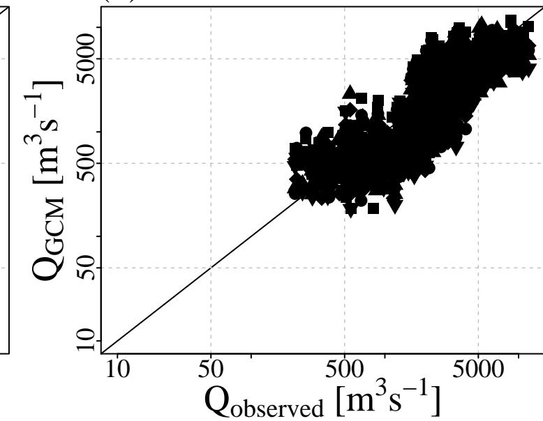
(d) MAX Observed vs. GCMs
