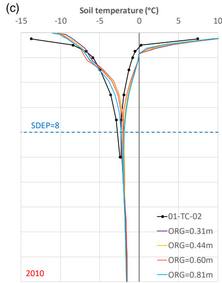
HPC – M-org (TBOT=-1.5°C)
