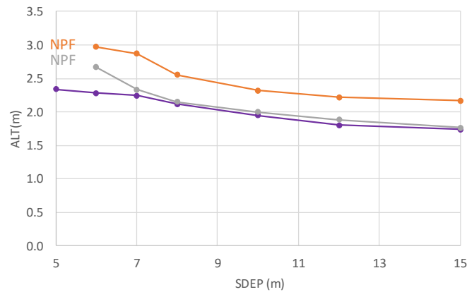
JMR – NL forest (ORG 1.46m, TBOT=+0.80°C)
