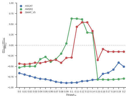
(d) Mississippi flood plain
