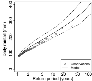
egp-(2,3)
