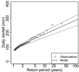
eexp-(2,3)
