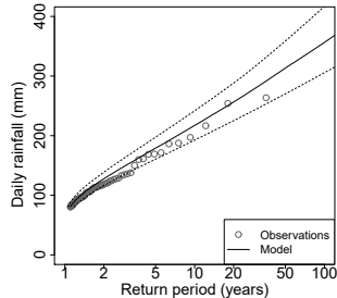
wei-(2,3)
