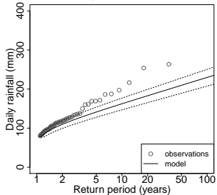
gamma-(1,1)
