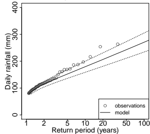
gamma-(2,1)
