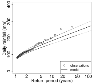
gamma-(1,3)
