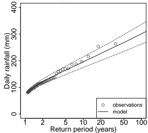
gamma-(2,3)
