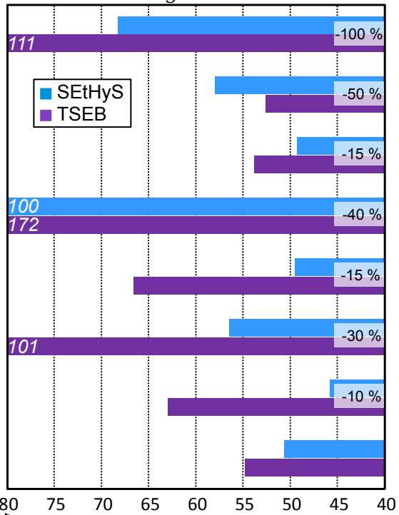
Resulting LE RMSE [W m 2 ]
