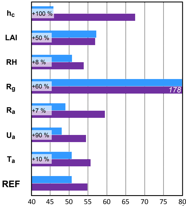
Resulting LE RMSE [W m 2 ]
