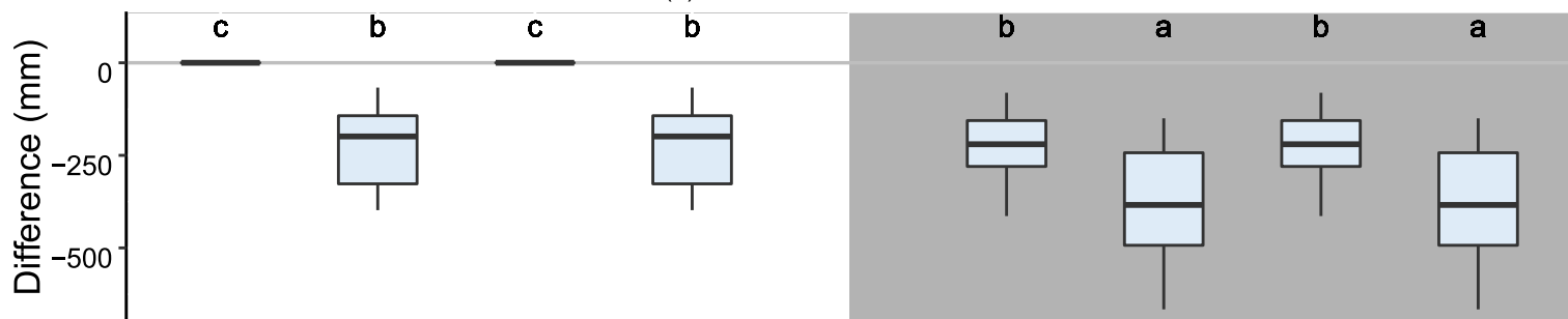
(d) Peak SWE: sink
