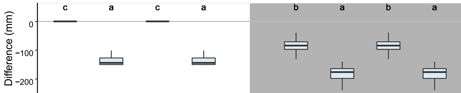
(d) Peak SWE: treeline
