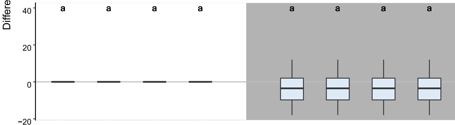
(d) Annual runoff
