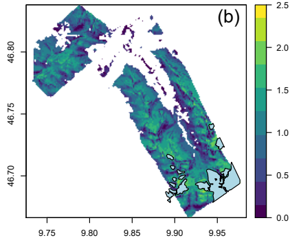
Posterior median
