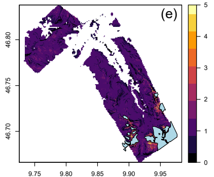
Posterior 90Q
