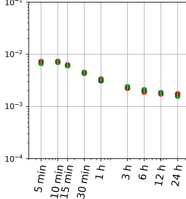
(d) RMSE
