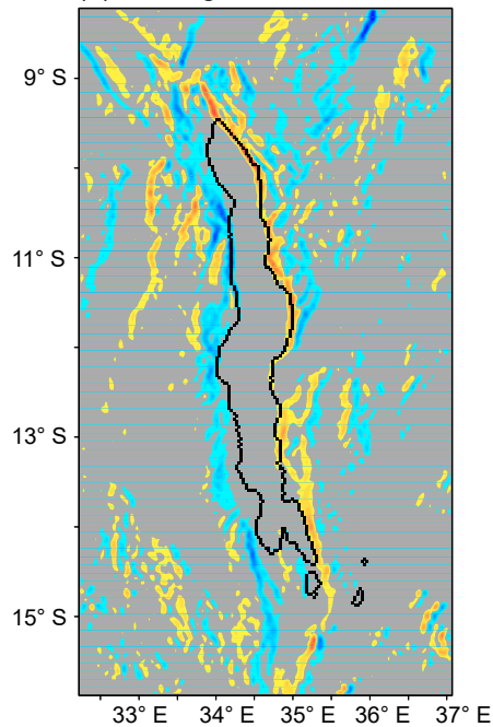
(b) Zonal gradient
