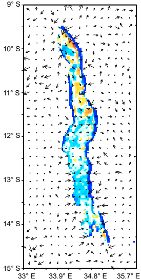
(b) WRF-NOLM
