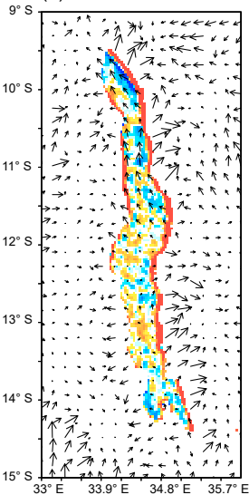
(e) WRF-NOLM
