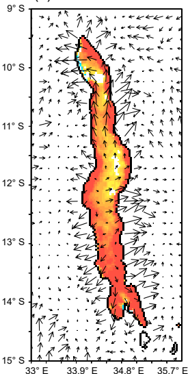
(d) WRF-CTL
