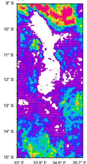
(e) WRF-NOLM
