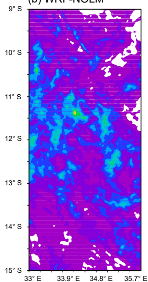
(b) WRF-NOLM
