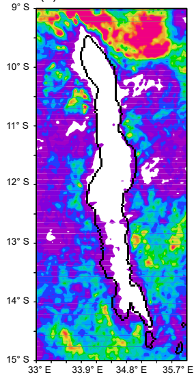
(d) WRF-CTL
