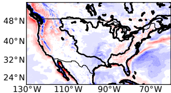
(d) T799 - T159
