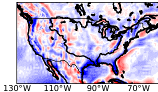
(e) T799 - ERAI
